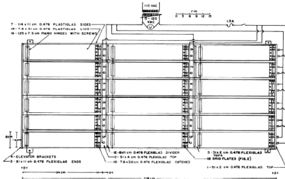
شکل ۳_ نمای فوقانی تردمیل بادنه‌انسن و جانسون (۱۹۷۱)
